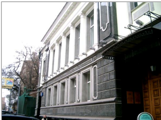
Фасад олимпийского комитета Гранит Хибинит, Мансуровский, Nero Zimbabwe Дизайн-проект И. Бирун-Орлов (КАМ)
